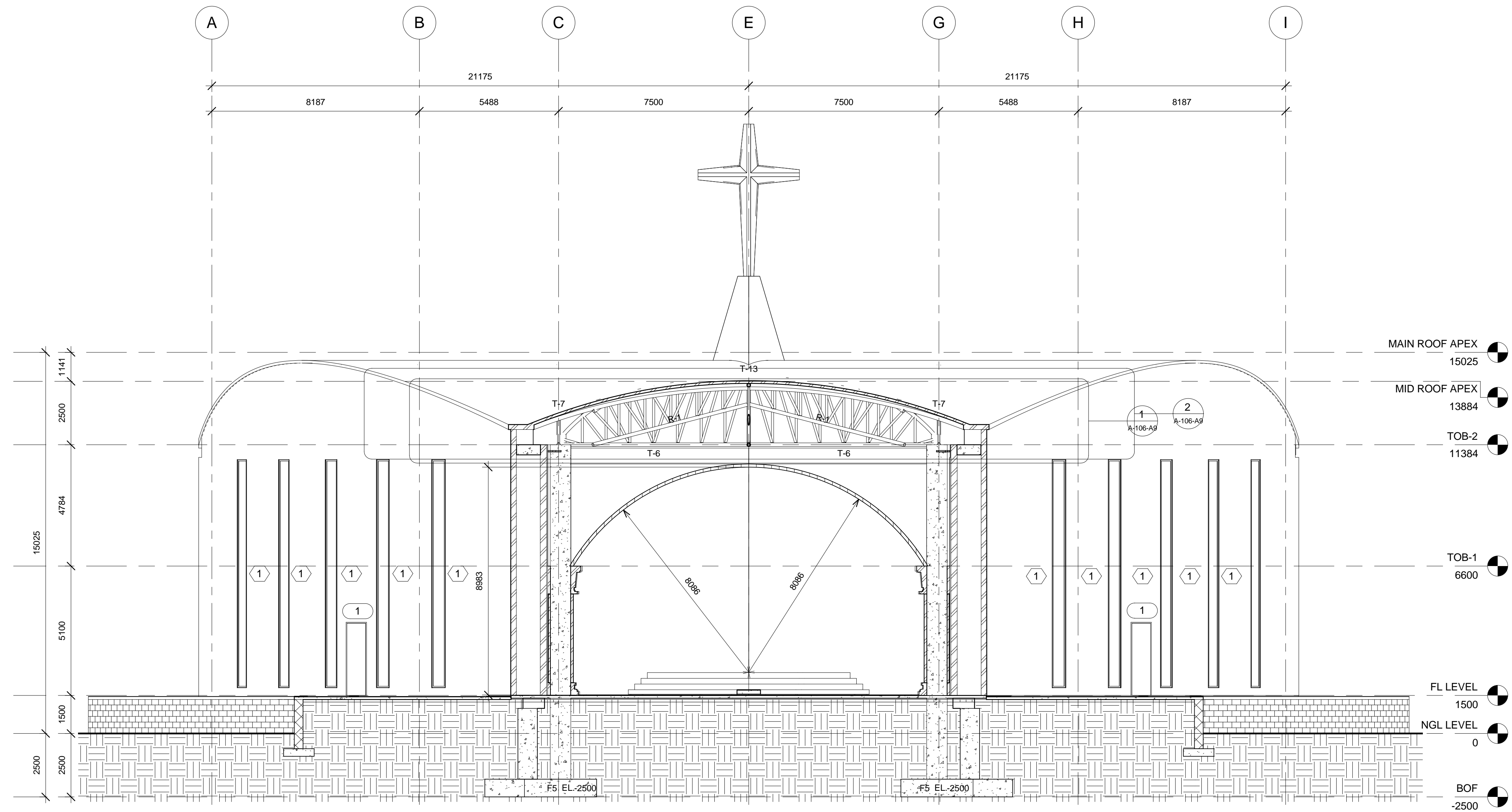
1 CROSS SECTION A 1 : 100
